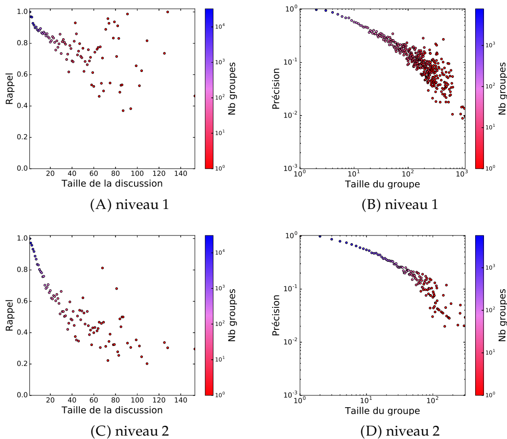
FIGURE 3.15 – (A,C) Rappel des discussions vis-à-vis des groupes trouvés par Louvain à différent niveaux récurifs. (B,D) Précision des groupes trouvés vis-à-vis des discussions. Chaque point représente la moyenne du rappel (resp. précision) pour les discussions (resp. groupes) ayant la même taille. La couleur du point indique le nombre de groupes ayant la même taille.
