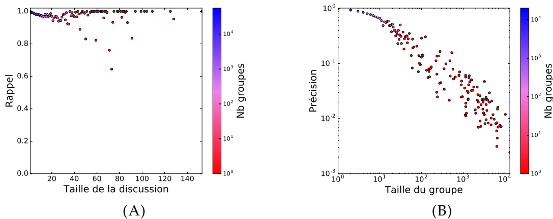
FIGURE 3.14 – (A) Rappel des discussions vis-à-vis des groupes trouvés par Louvain. (B) Précision des groupes trouvés vis-à-vis des discussions. Chaque point représente la moyenne du rappel (resp. précision) pour les discussions (resp. groupes) ayant la même taille. La couleur du point indique le nombre de groupes ayant la même taille.
