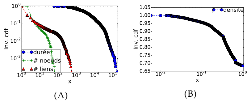
FIGURE A.9 – Distribution cumulative inverse du nombre de liens, de noeuds et de la durée en (A) et de la densité en (B) pour les candidats trouvés par la méthode de Louvain dans le jeu de données Reality Mining.
