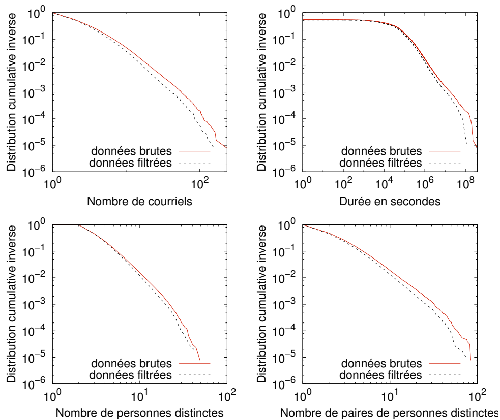
FIGURE 3.1 – Distribution cumulative inverse de différentes caractéristiques des données brutes (ligne pleine) et filtrées (ligne en pointillé). En haut à gauche : nombre de courriels dans une discussion ; en haut à droite : durée d’une discussion ; en bas à gauche : nombre de personnes dans une discussion ; en bas à droite : nombre de paires de personnes en interaction distinctes dans une discussion.
