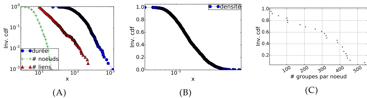
FIGURE A.8 – Distributions cumulatives inverses du nombre de liens, de noeuds et de la durée en (A), de la densité en (B), du nombre de groupes par noeud en (C) pour les groupes capturés par notre méthode dans les données Babouins.
