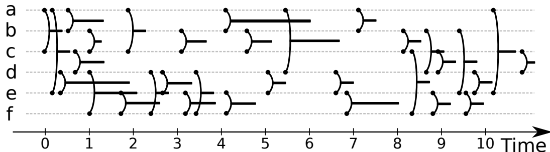
FIGURE 1.6 – Flot de liens entre 6 nœuds ( en ordonnées) au cours du temps (en abscisses). Dans l'exemple, il existe un lien entre a et b durant l'intervalle [4, 6] .
