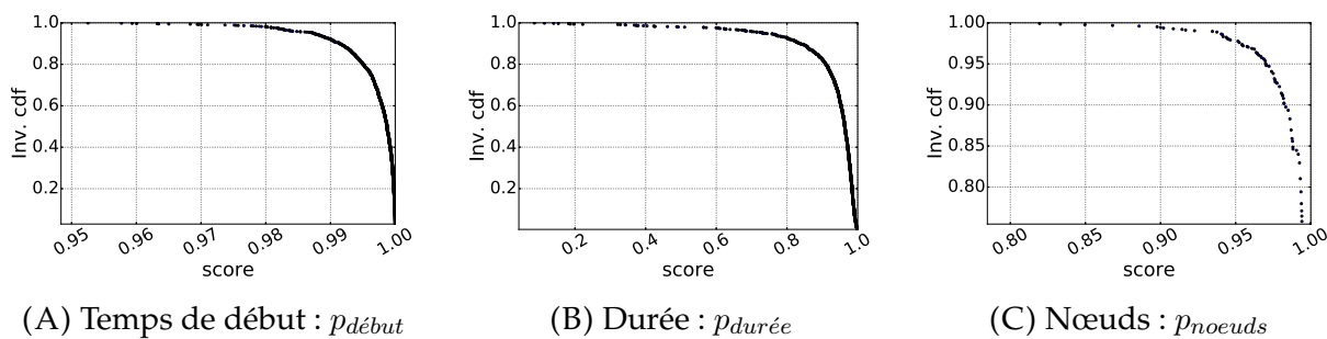
FIGURE A.6 – Distribution cumulative inverse des scores pour chaque voisinage dans le jeu de données Babouins.
