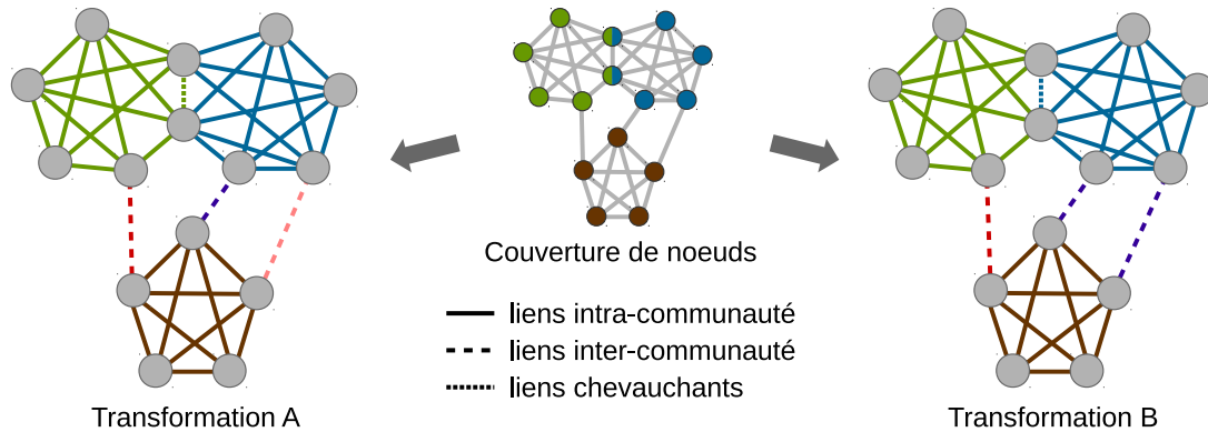
FIGURE 5.12 – Construction de TA et TB depuis une couverture de noeuds. La couleur des liens indique leur groupe.
